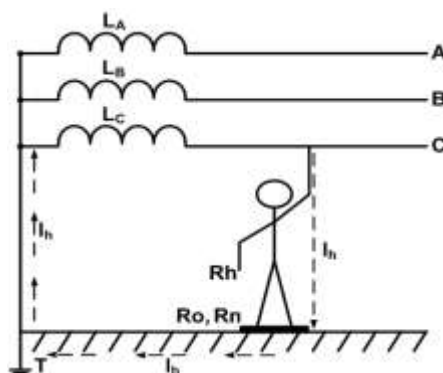
Рис. 1.4. Однополюсное прикосновение человека к неповрежденной 3-фазной сети с глухозаземленной нейтралью
