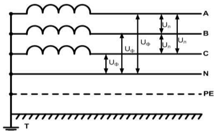
Рис. 1.2. Пятипроводная 3-фазная сеть переменного тока с глухозаземленной нейтралью, нулевым рабочим N и защитным PE проводниками
